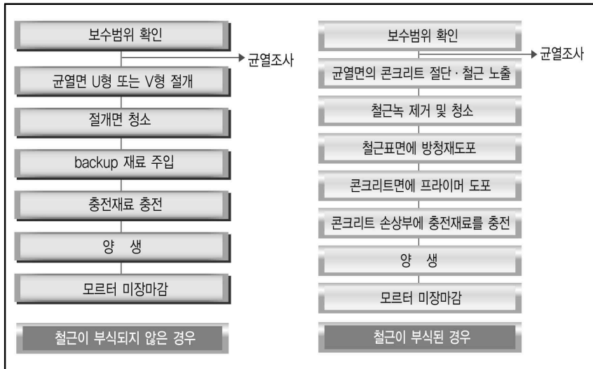
[균열 보수(충전공법) 시공 순서도]
