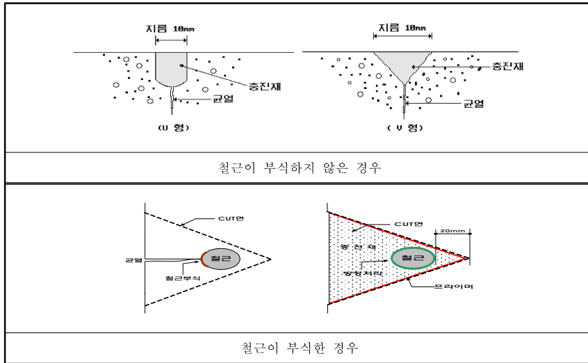
[균열 보수(충전공법) 개념도]
