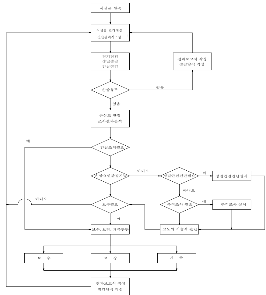
[유지관리 흐름도]
