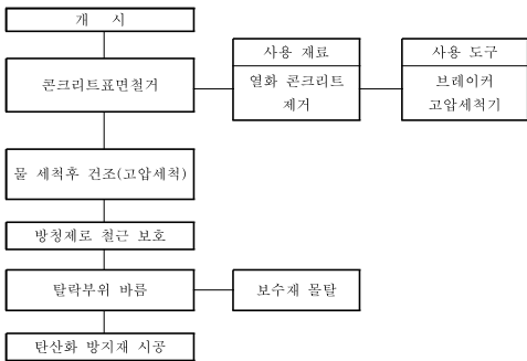
[단면복구공법 시공순서도]
