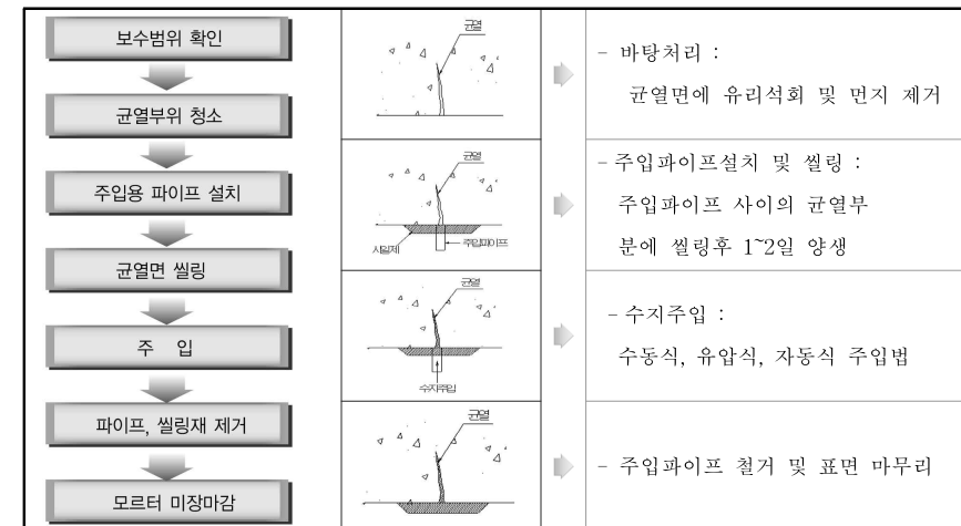
[균열 보수(주입공법) 시공 순서도 및 상세도]
