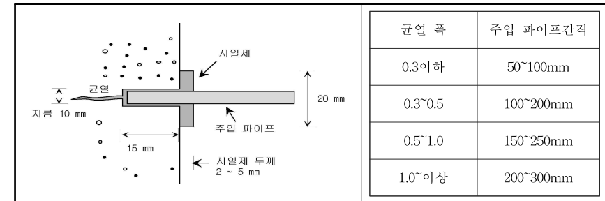
[균열 보수(주입공법) 개념도]
