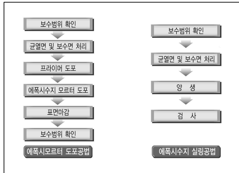
[균열보수 (표면처리) 시공 순서도]
