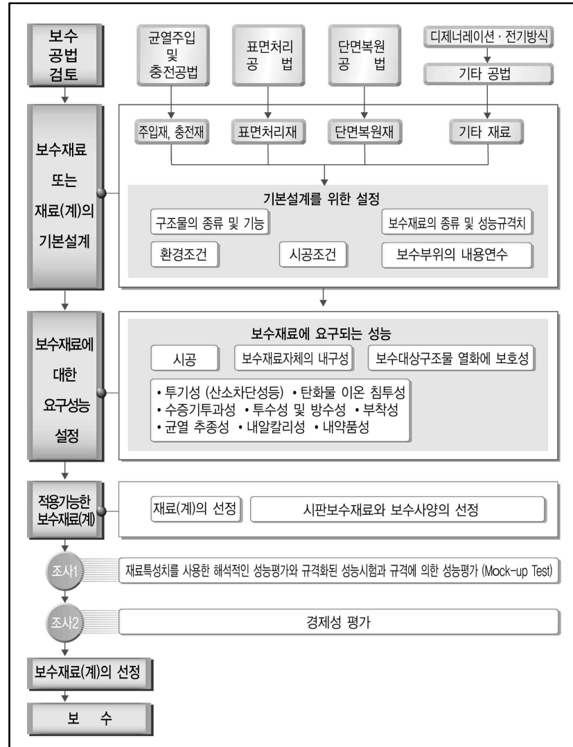
[보수재료 선정 흐름도]
